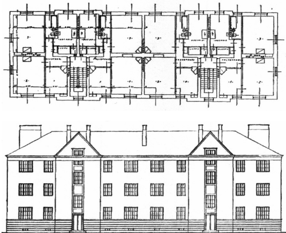
Rzut piętra oraz elewacja wejściowa domu dla oficerów przy ul. Kościuszki 20 w Kutnie. Źródło: „Architektura i Budownictwo” 1929, nr 2-3, s. 6
