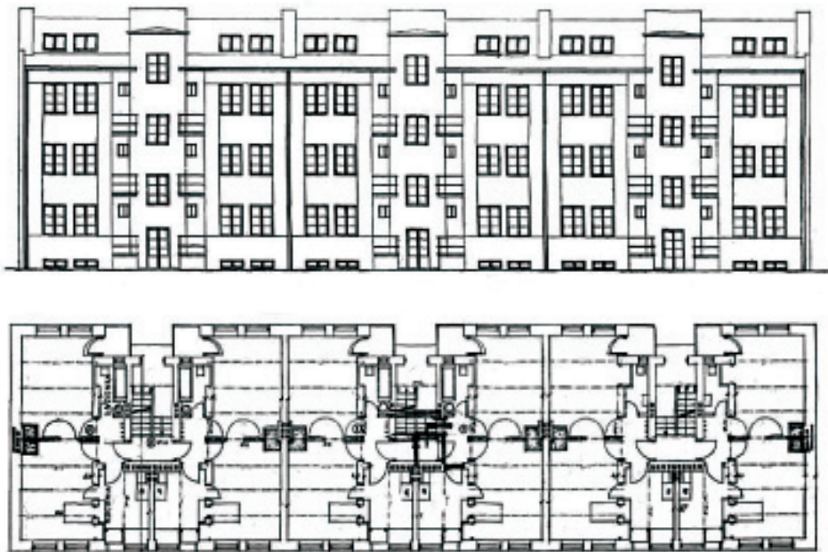
Rzut parteru i elewacja wejściowa domu dla podoficerów przy ul. Ułańskiej 2 w Płocku. Źródło: „Architektura i Budownictwo” 1929, nr 2-3, s. 61.
